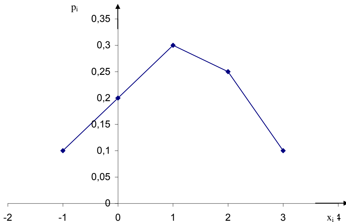
Многоугольник распределения
